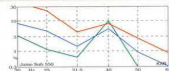
Harmoninen särö (THD) 80 dB (vihreä), 90 dB (sininen) ja 100 dB (punainen) tasolla.
