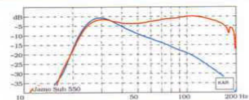
Vapaakenttäväte jakosuotimen ääriarvoissa.
